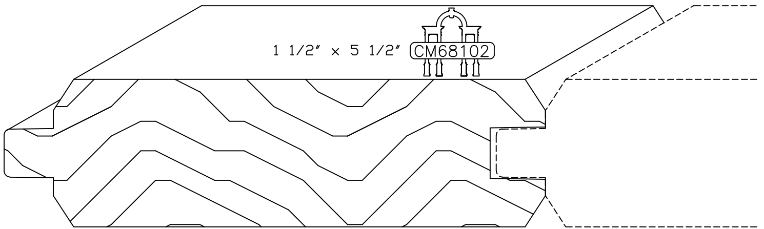
V-JOINT T&G
